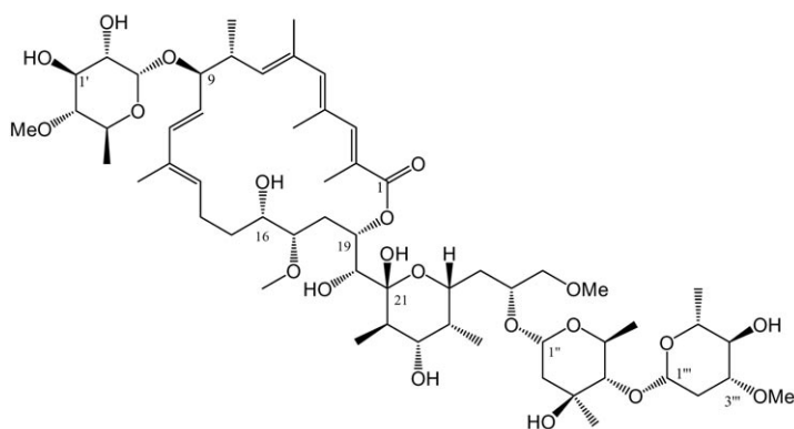
Apoptolidin
